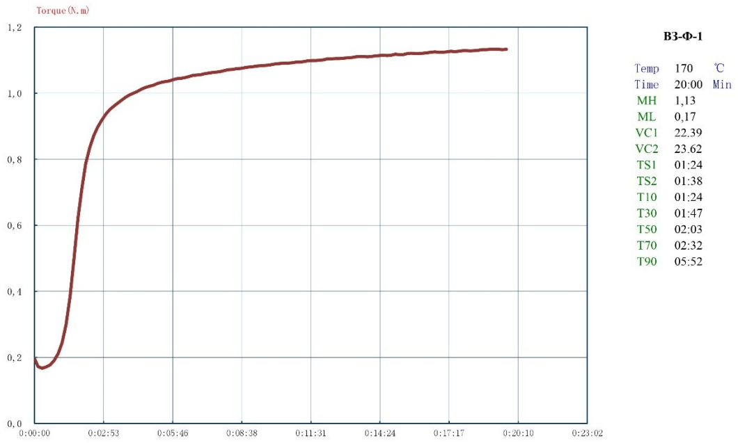
Вулканизационная кривая резиновой смеси ВЗ-Ф-1
